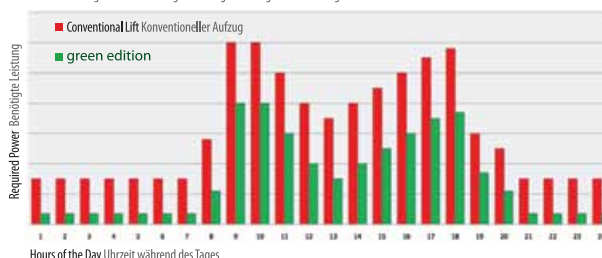
Sample diagram: Power required from an office building lift Indikatives Diagramm der benötigten Aufzugs-Leistung in einem Bürogebäude
